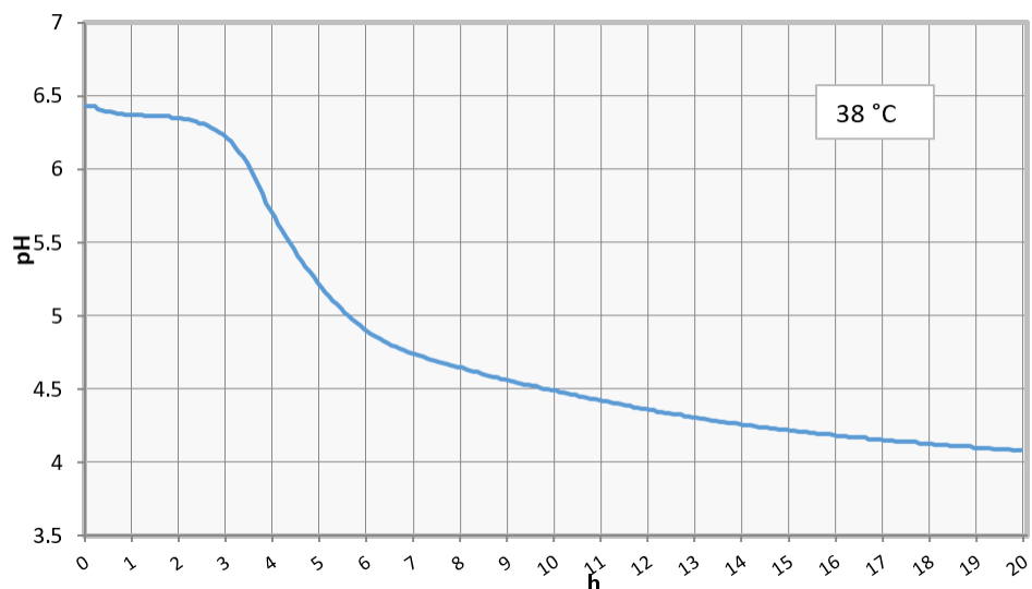
Milieu: poudre de lait maigre reconstitué, stérilisé. Quantité d'ensemencement: 1 ‰ température d'incubation: 38°C
